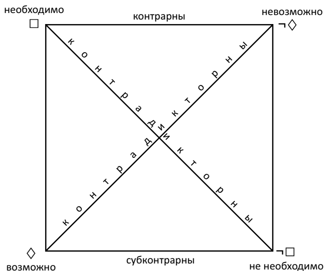
Рис. 1. Логический квадрат алетической модальности
